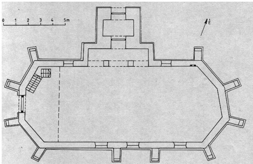
Méhtelek. Református templom alaprajza.
